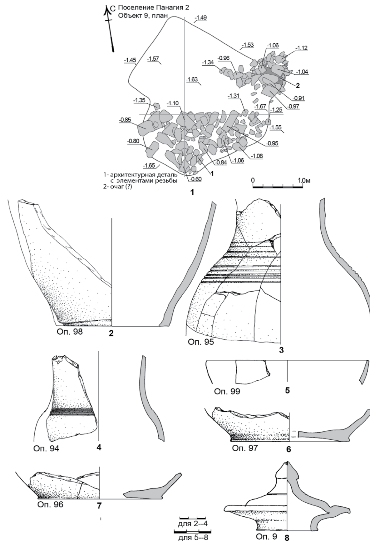
Рис. 1. Поселение Панагия 2, объект 9: 1 – план полуземлянки; 2–8 – фрагменты керамических сосудов из заполнения
